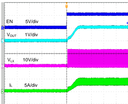
Startup from EN
