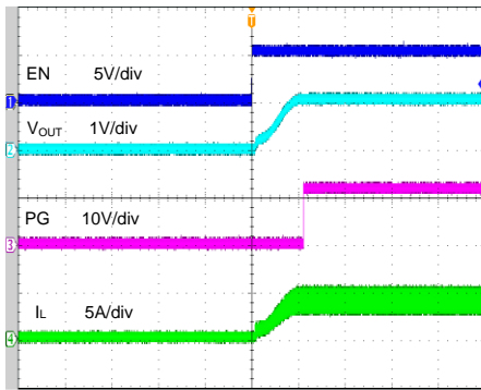
PG Test (EN On) ( V_{IN}=12V , V_{OUT}=1.05V , I_{OUT}=4A )
