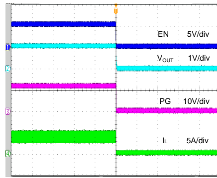
PG Test (EN Off) ( V_{IN}=12V , V_{OUT}=1.05V , I_{OUT}=4A )
